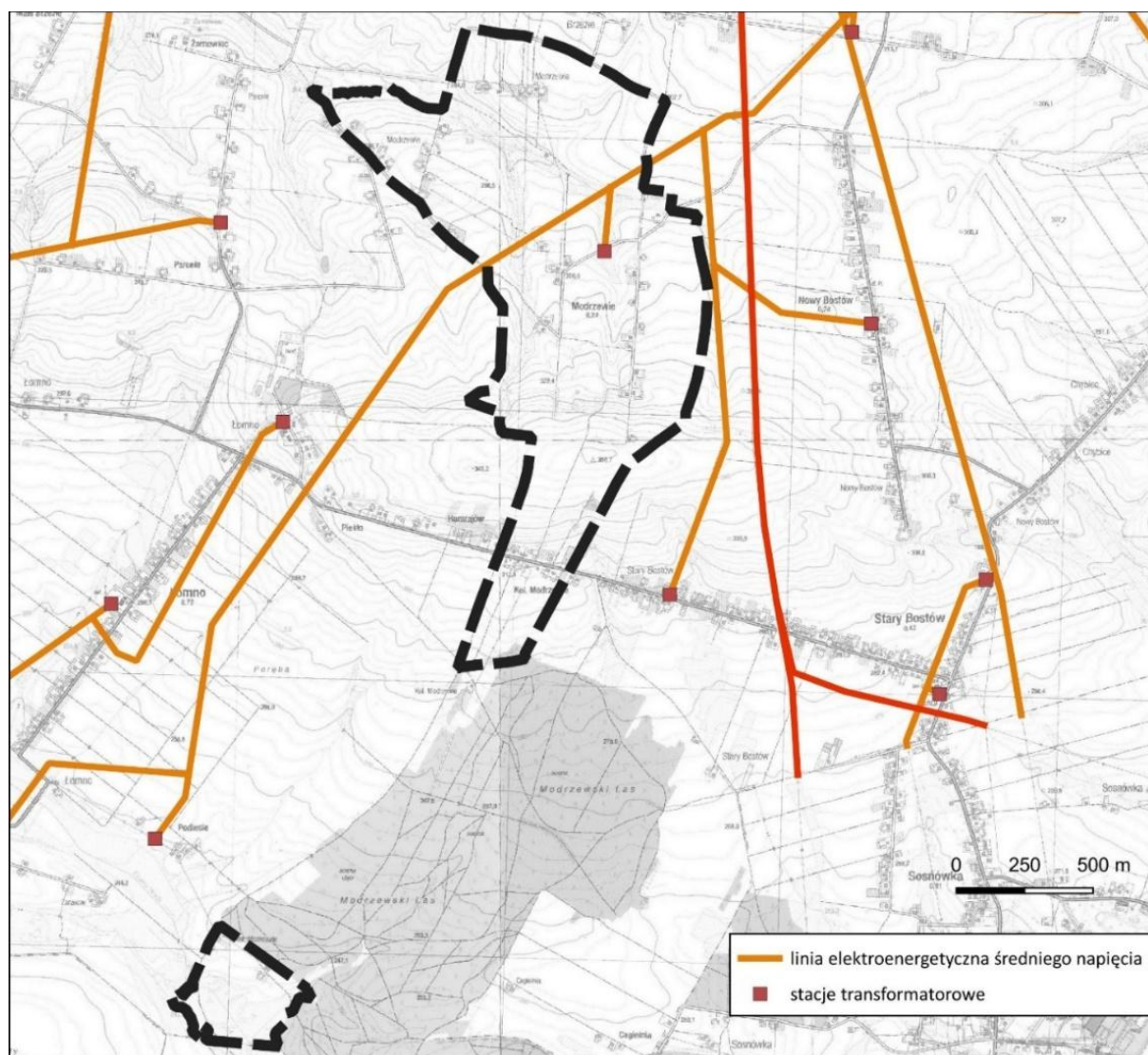
Rysunek 11. Przebieg linii elektroenergetycznych na terenie opracowania
